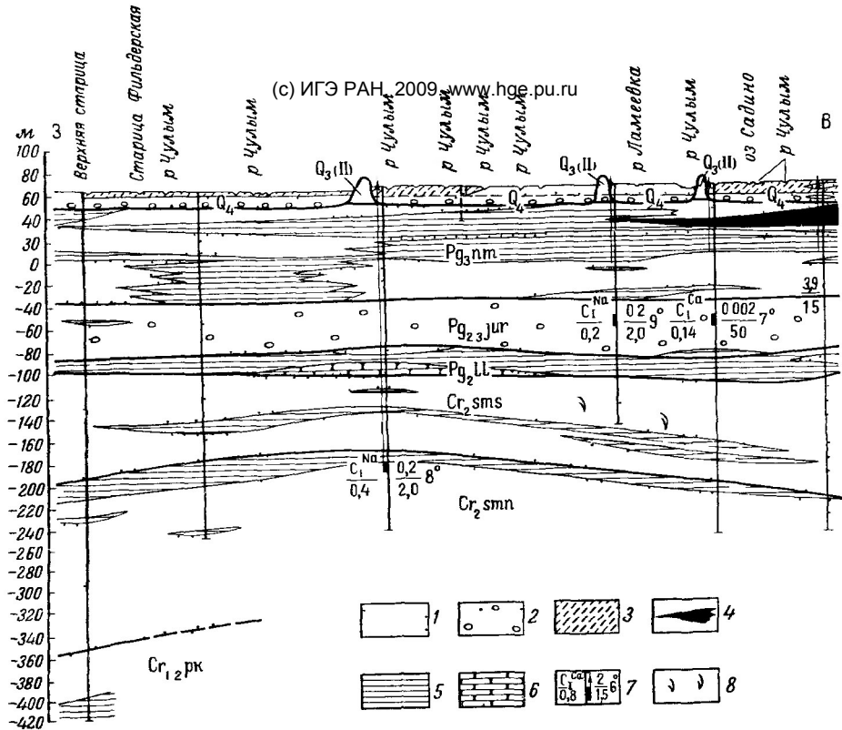
Рис. 14. Схематический гидрогеологический разрез вдоль р. Чулым (по Л. К. Чагиной, 1964)
