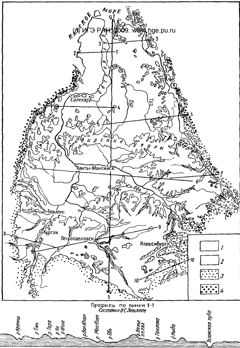
Рис. 1. Схематическая гипсометрическая карта (составили Н. А. Мошкина и А. Н. Храмова) Высоты, м 1 — до 100, 2 — от 100 до 200; 3 — от 200 до 400, 4 — 400—600 и выше
