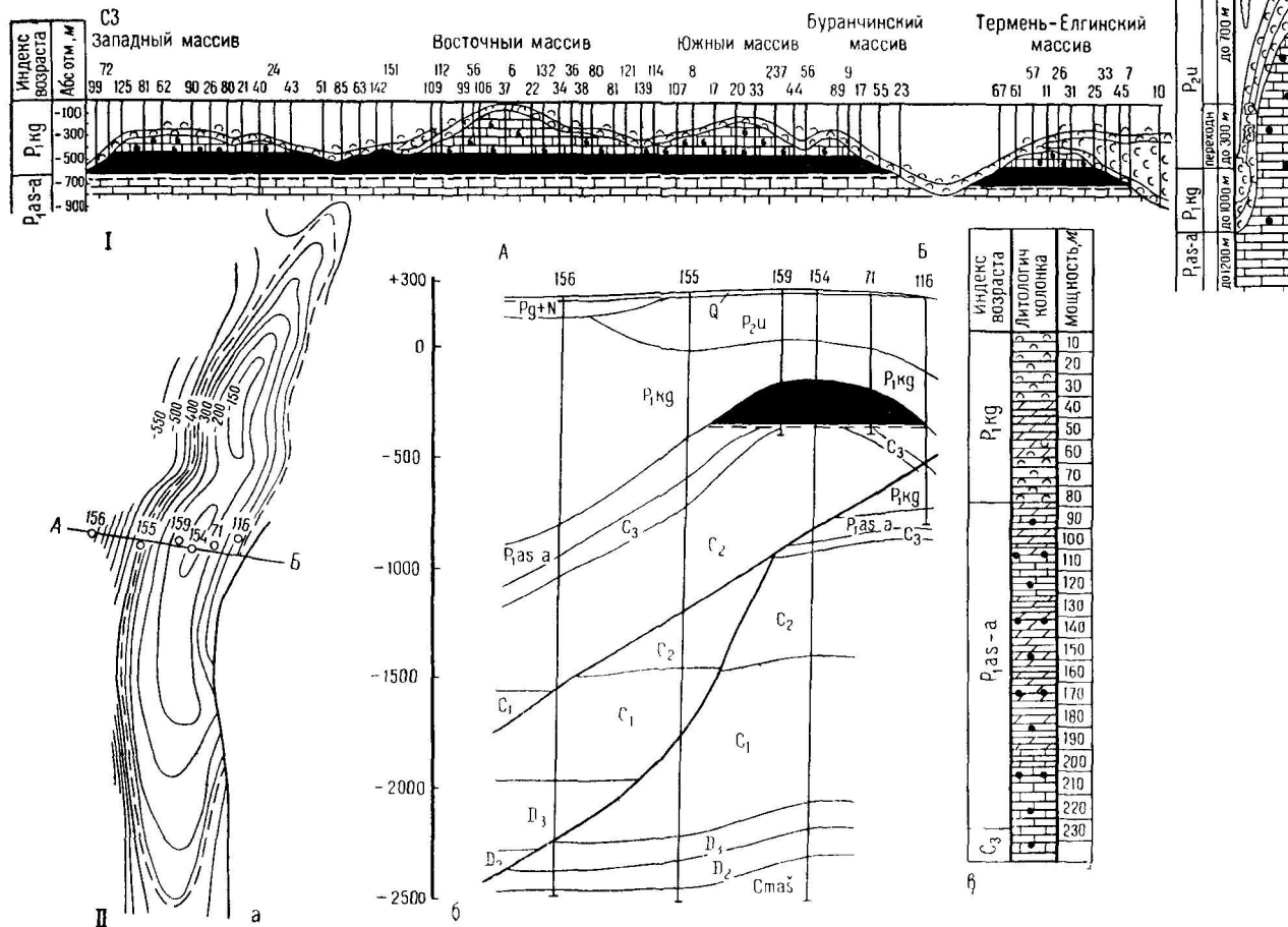
Рис. 31. Схема строения Ишимбайской группы (I), газо-нефтяных месторождений и Кинзебулатовского месторождения (II) (по Д. Ф. Шамову и др.): а — структурная карта по кровле артинских отложений; б — геологический профиль; в — сводная геологическая колонка. Условные обозначения см. на рис. 29
