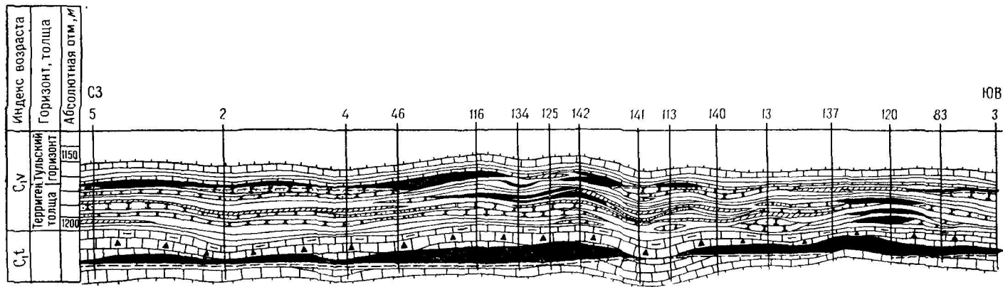
Рис. 30. Схема строения Манчаровской группы нефтяных месторождений. Разрез залежей нижнего карбона (по И. Л. Зубику)
