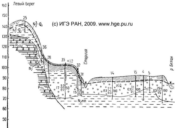
Рис. 19. Гидрогеологический разрез левобережной части долины р. Белой в районе г. Уфы. Составил М. С. Верзаков Условные обозначения см. на рис. 18.
