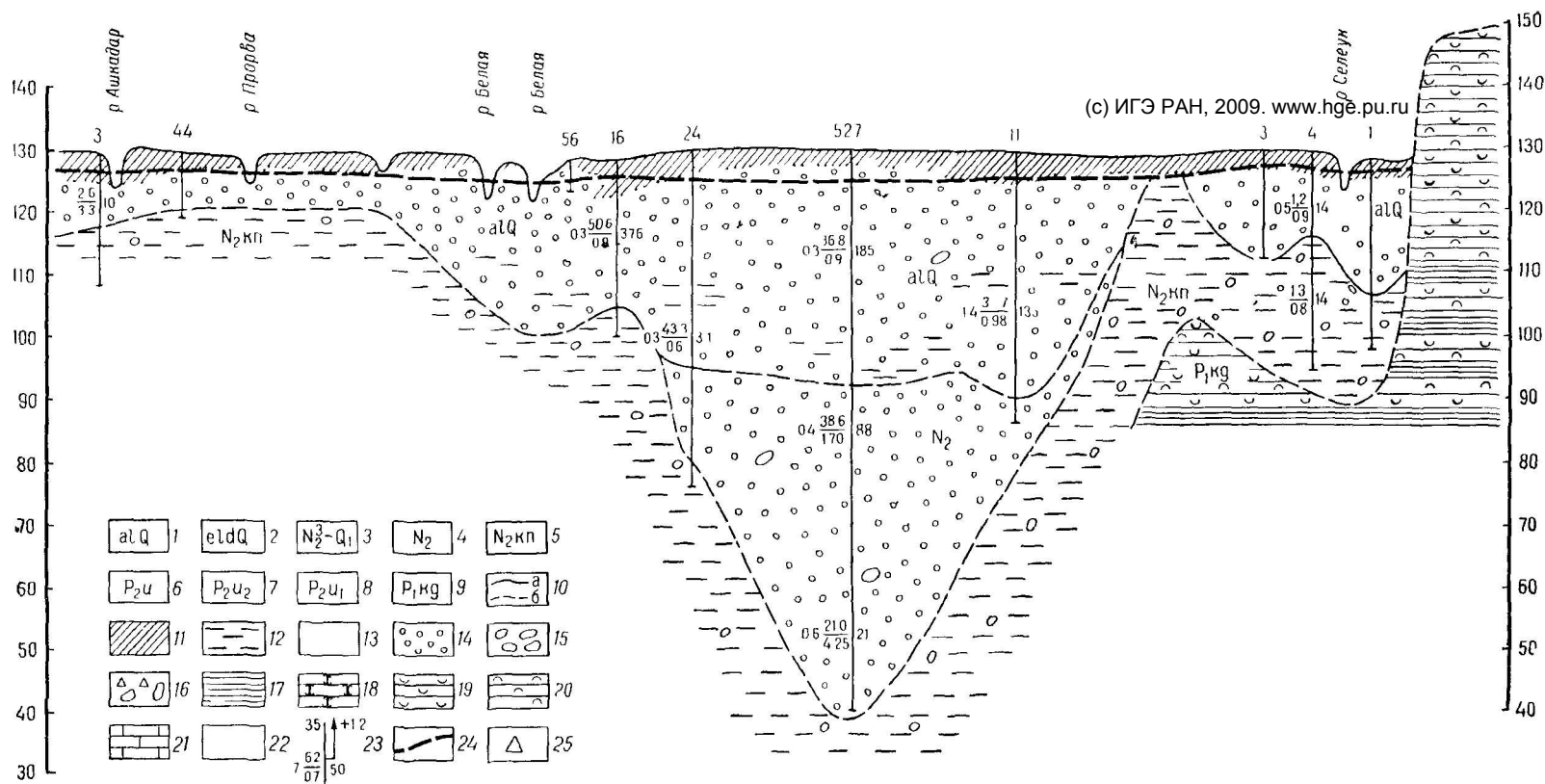
Рис 18 Гидрогеологический разрез через долину р. Бетой в районе г. Стерлитамака (по И. М. Загородневой и В. А. Дубровскому, 1961)
