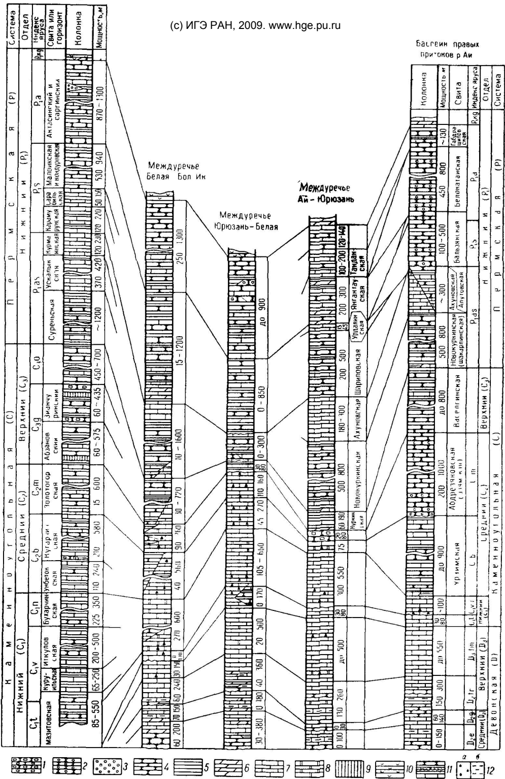
Рис. 13. Схема сопоставления разрезов нижнепермских (докунгурских), каменноугольных и девонских отложений восточного борта Предуральяского прогиба и Западно-Уральской внешней зоны складчатости (по данным А. Э. Алкснэ, Г. А. Смирнова, З. А. Синициной, И. И. Синицына, С. Н. Краузе, А. П. Тяжевой и др.)
