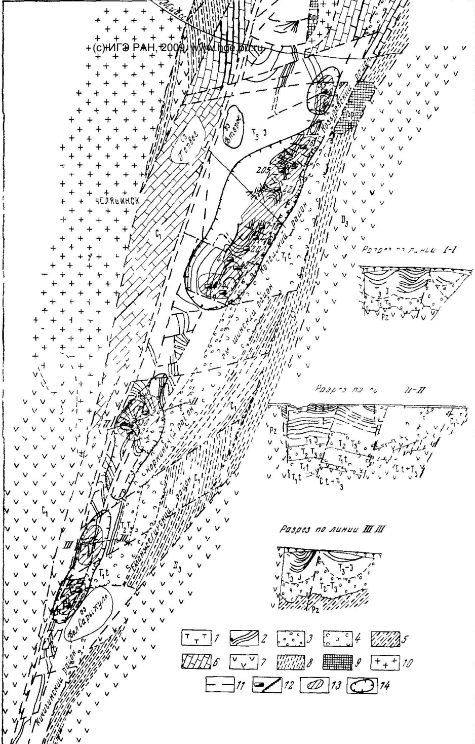
Рис. 106. Геолого-тектоническая и гидрогеологическая схема Челябинского бурогоугольного бассейна (покров мезо-кайнозойских пород на схеме снят). Составили В. И. Антипин, А. П. Сирман по материалам разведочных работ
