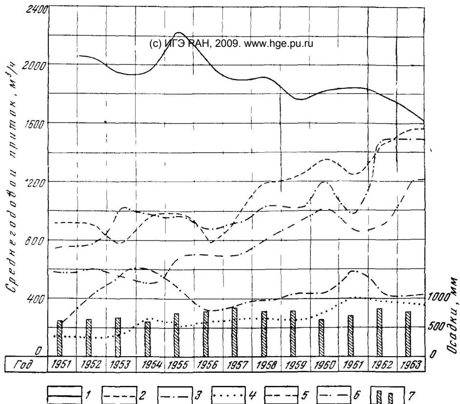
Рис 99. График изменения среднегодового притока подземных вод в шахты Кизеловского каменноугольного бассейна. Составил Ю. А. Ежов
