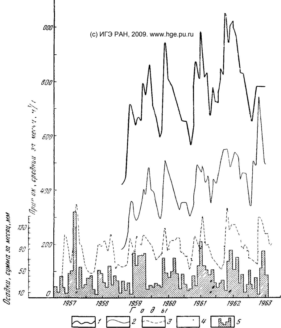
Рис 96 График водопритоков Баженовского месторождения хризотил-асбеста По М. М. Трапезниковой и В. М. Чемякину
