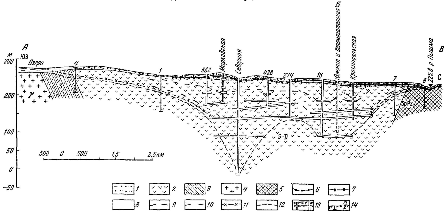
Рис. 95 Гидрогеологический разрез жильного поля Берзовского золоторудного месторождения Составила Л. С. Архангельская по материалам Уралгидростанции за 1956 г
