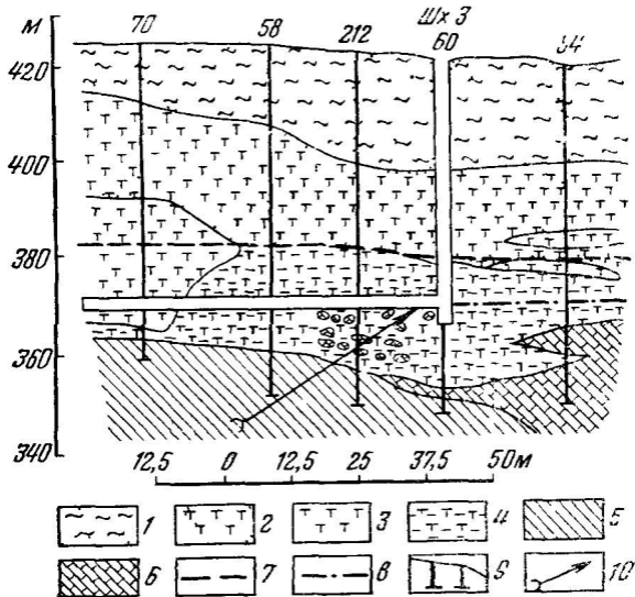
Рис 93 Гидрогеологический разрез Шелеинского месторождения никеля
