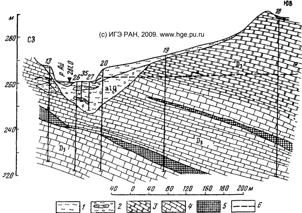
Рис 91. Гидрогеологический разрез Блиново-Каменского месторождения бокситов (по материалам Уралгидростанции)
