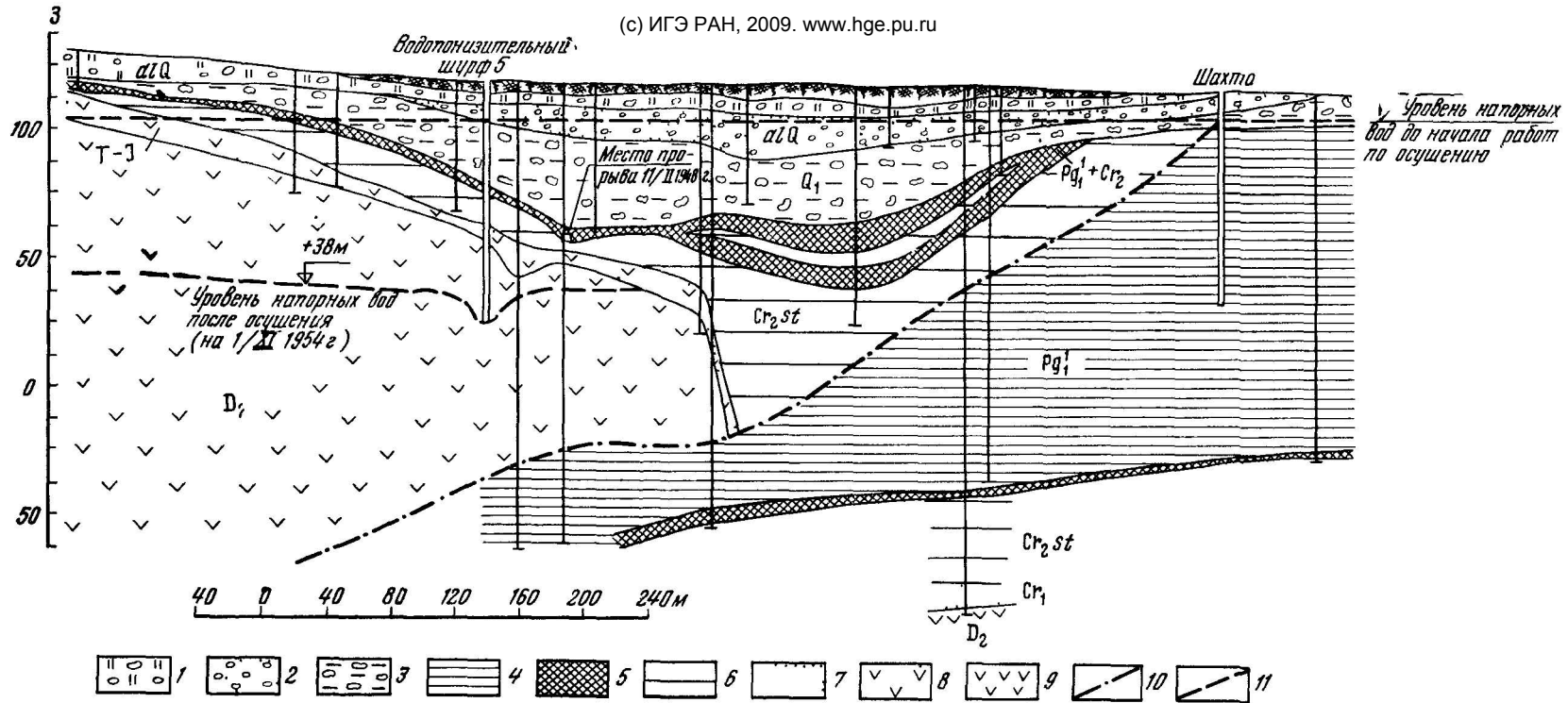
Рис 88 Гидрогеологический разрез Полуночного месторождения (в районе прорыва подземных вод). По Н С Шабалиной
