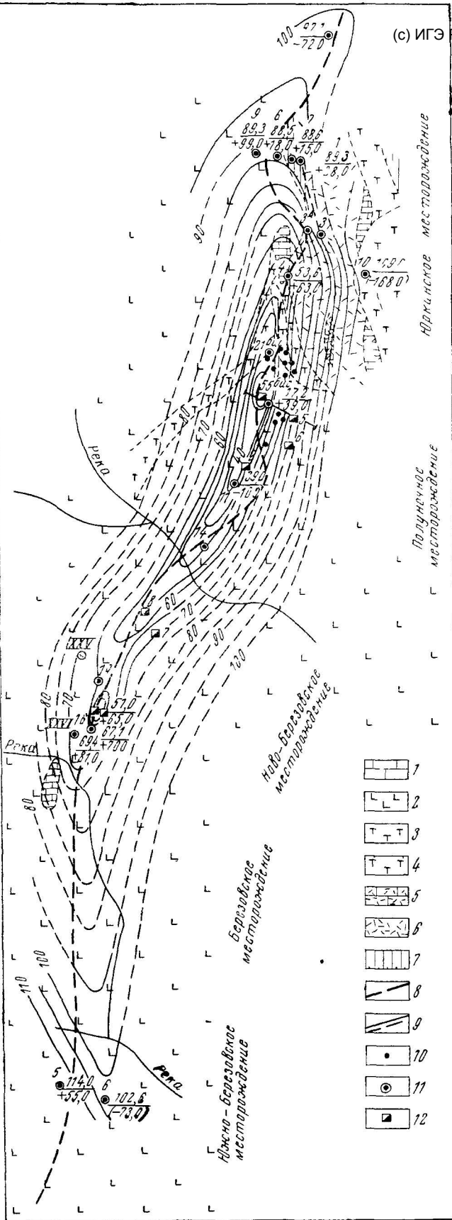
Рис. 87. Карта гидроизопьез водоносного комплекса зон трещиноватости вулканогенно-осадочных пород по Северной группе марганцевых месторождений: Юркинскому, Полуночному и Березовским. По Н. С. Шабалной
