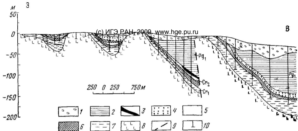
Рис 86. Схематический широтный разрез Марсятского (железорудного и марганцевого) месторождения. По И. А. Пайтелеву и А. И. Краевой
