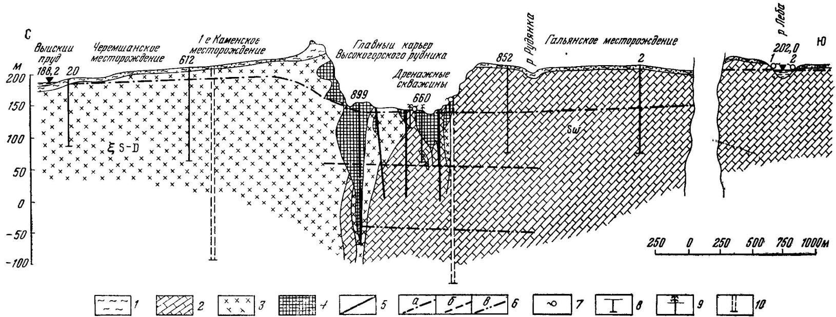
Рис 84 Гидрогеологический разрез Высокогорского железорудного месторождения (по простиранию Главной рудной зоны). Составила Л. С. Архангельская по материалам М. Я. Барабашкина и Уралгидростанции 1 — аллювиальные и делювиальные песчано-глинистые отложения 2 — известняки 3 — сиениты, 4 — железорудная толща, 5 — линии тектонических нарушений, 6 — динамический уровень подземных вод а — на 1/X 1953 г., б — на 1/I 1961 г., в — 1/I 1966 г., 7 — родники, 8 — скважины, 9 — фонтанирующая скважина (1953 г.), 10 — шахты
