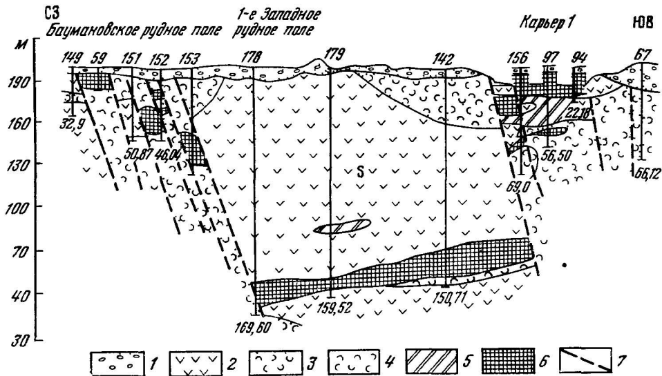
Рис 83 Геологический разрез Покровского железорудного месторождения По М Я Бара башкину
