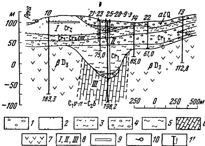
Рис 78 Гидрогеологический разрез придолинного месторождения подземных вод смешанного типа в малой депрессии Тобольского артезианского бассейна III-7-A 2 -б. Составила А. С. Веретенникова по материалам К. А. Костиной и Я. Я. Сердюка
