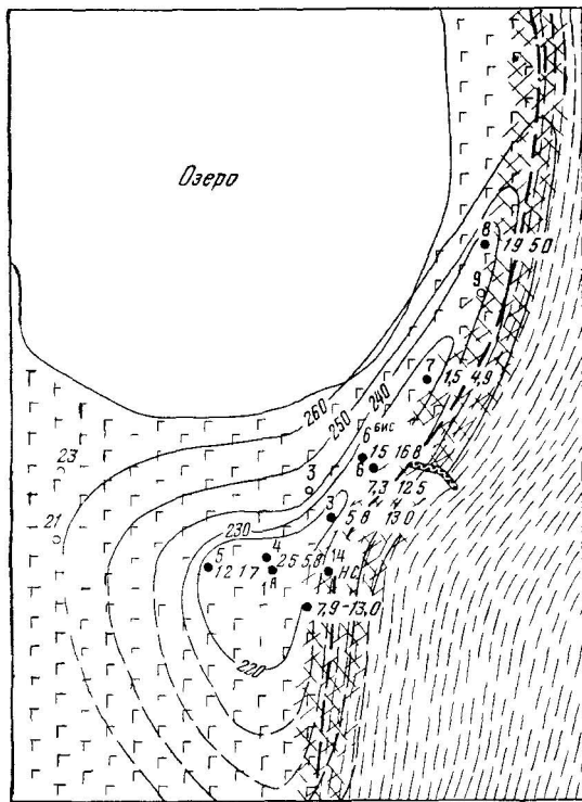
Рис. 76. Схематическая гидрогеологическая карта придолинного месторождения трещинно-жильных вод, приуроченного к зоне тектонического контакта, III-6-A 2 -б 1 . Составили А. С. Веретенникова и Н. А. Евсева по материалам Уралгидростанции
