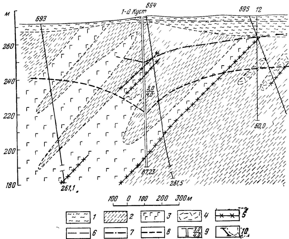
Рис. 75. Гидрогеологический разрез придолинного месторождения трещинно-жильных вод III-6-А 1 -а 2 . Составил А. С. Веретеникова по материалам А. А. Хмелевского
