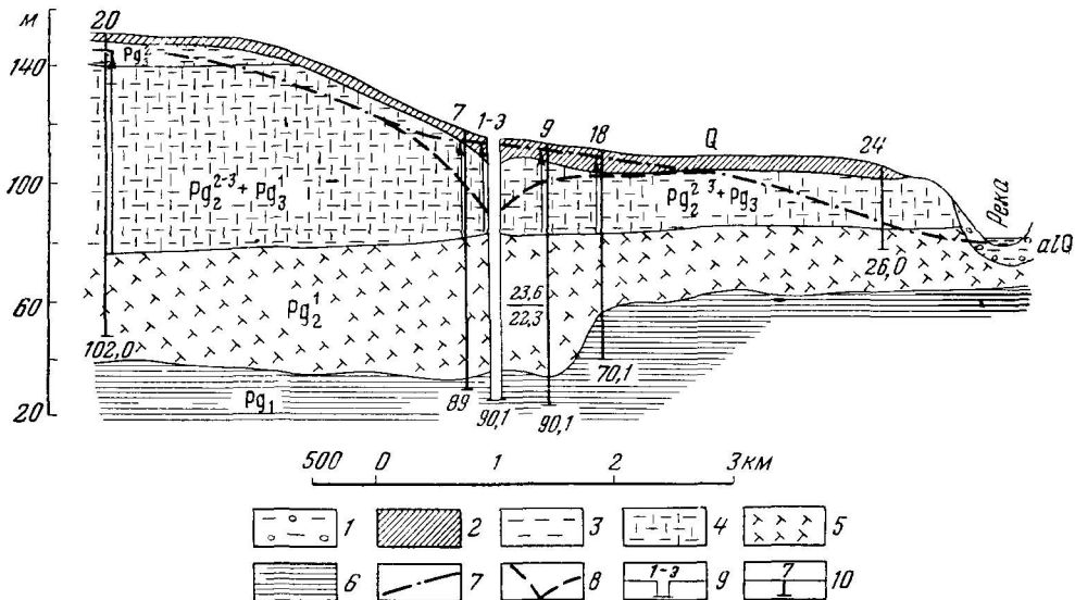
Рис. 72. Меридиональный гидрогеологический разрез водораздельного месторождения пластово-трещинных вод II-4-Б 1 -Б 2 . По материалам А. С. Веретенниковой
