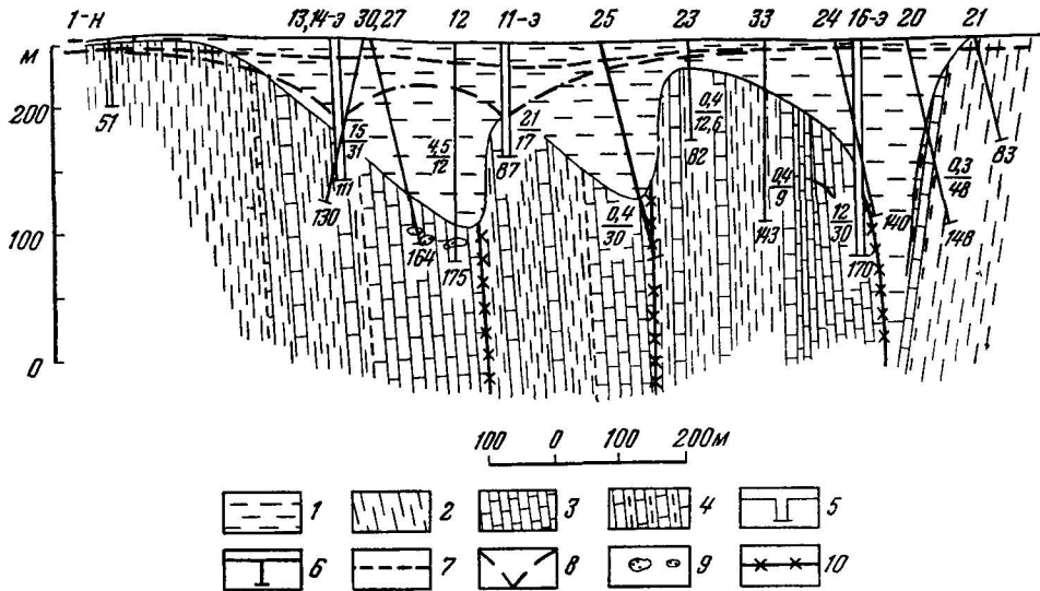
Рис 71 Гидрогеологический разрез водораздельного месторождения напорных трещинно-карстовых вод в малом массиве карбонатных пород II-3-B 2 . Составила А С Веретенникова по материалам М А Фаденчевой
