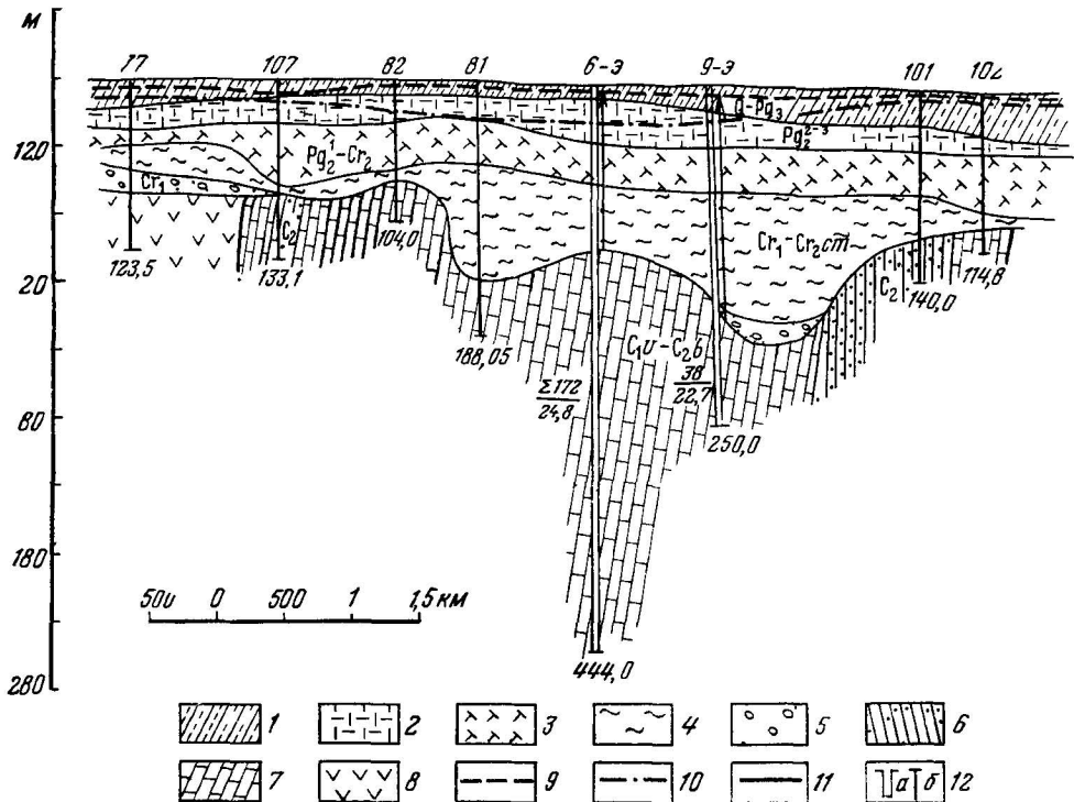
Рис. 70. Гидрогеологический разрез водораздельного месторождения напорных трещинно-карстовых вод в крупном карбонатном массиве П-3-Б 1 -б 2 . По материалам А. С. Веретенниковой
