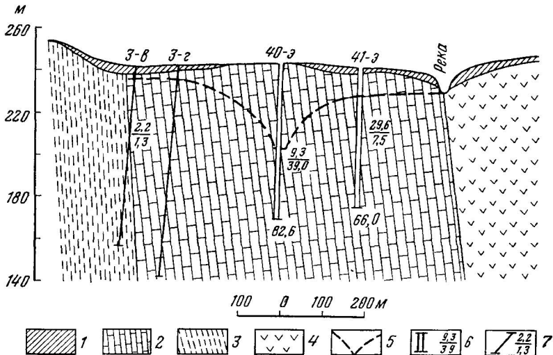
Рис. 68. Гидрогеологический разрез придолинного месторождения трещинно-карстовых вод в малом карбонатном массиве — I-3-A 2 -а, Составила А. С. Веретенникова по материалам А. К. Костиной
