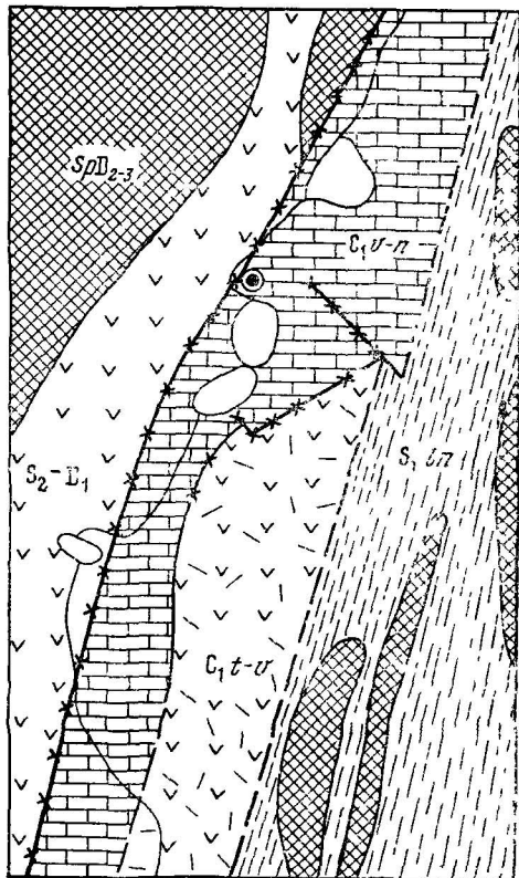
Рис. 67. Схематическая гидрогеологическая карта придолинного месторождения трещинно-карстовых вод в крупном карбонатном массиве, осложненном блоковой тектоникой 1-3-А 1 -а. Составила А. С. Веретенникова по материалам А. К. Муфтахова
