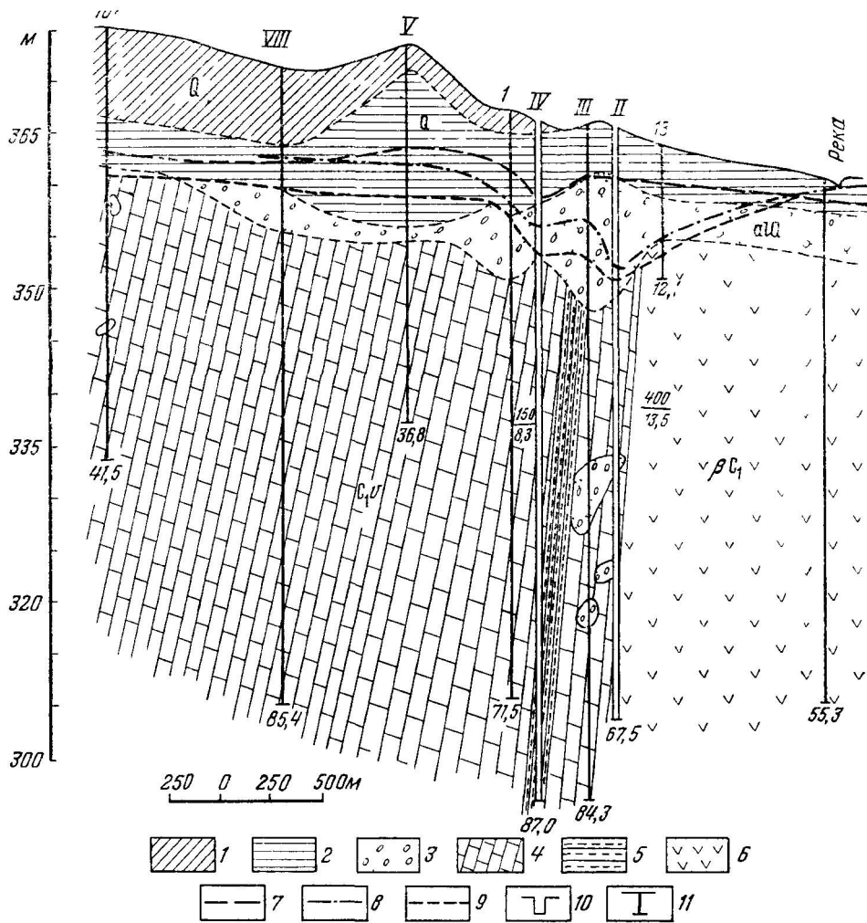
Рис. 66. Гидрогеологический разрез инфильтрационного месторождения трещинно-карстовых вод в крупных массивах карбонатных пород 1-3-А 1 -а 2 . По материалам Сирмана А. П. и Зайцева Г. И. 1 — суглинки; 2 — глины; 3 — песчано-гравелистый аллювий; 4 — известняки; 5 — аргиллиты, алевролиты, песчаники; 6 — порфириты и их туфы. Динамический уровень воды: 7 — до пробно-эксплуатационной откачки (1954 г.); 8 — на конец откачки (1955 г.); 9 — при эксплуатации на октябрь 1965 г., 10 — эксплуатационные скважины, 11 — поисково-разведочные и наблюдательные скважины. Цифры в числителе — среднемесячный расход скважины за октябрь 1965 г., в знаменателе — динамический уровень на этот же период.
