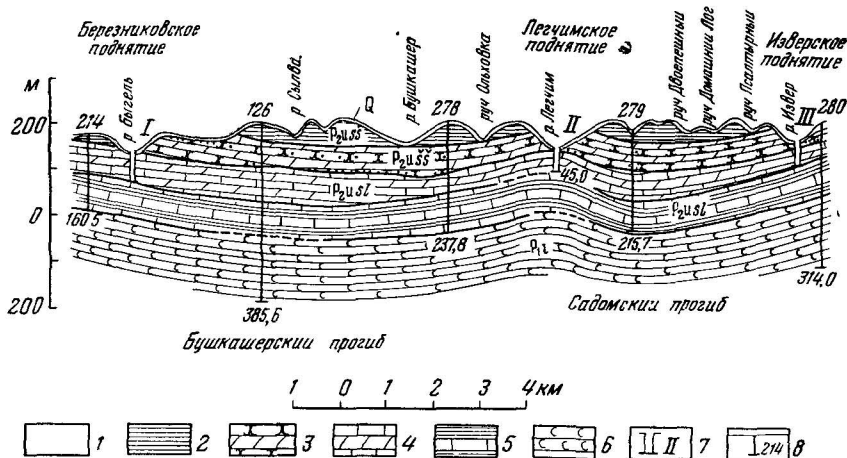
Рис. 65. Гидрогеологический разрез прилощинных месторождений трещинных вод Восточно-Русского артезианского бассейна в малых массивах некарстующихся пород I-2-A 2 -a 2 . По материалам Е. А. Боровиковой
