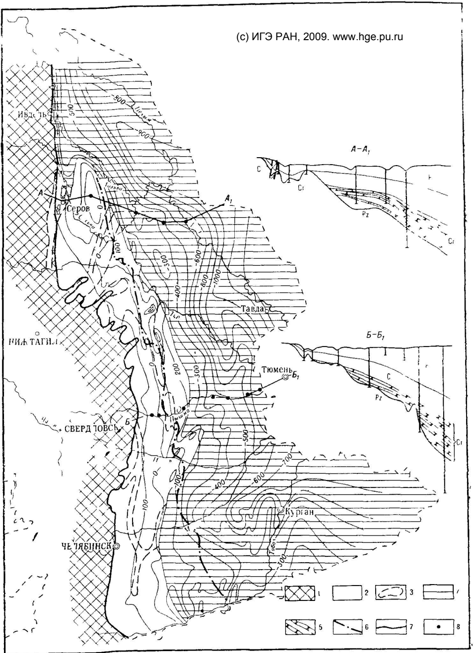
Рис. 54. Гидрогеологическая схема нижнемеловых отложений Зауралья Составил В. И. Антипин 1 — область распространения водоносных комплексов зон трещиноватости складчатого Урала, 2 — область нижнемелового континентального выветривания палеозойских пород фундамента. Воды распространены в зоне выветривания и локальных трещинных зонах, 3 — реликты нижнемеловых и сеноманских речных долин, выполненных водоносными аллювиальными отложениями (синарская и мысовская свиты); 4 — область распространения водоносного комплекса отложений нижнего мела (княгининская, викуловская, ханты-мансийская и уватская свиты); 5 — положение водоносного комплекса отложений нижнего мела в разрезах по линиям: А—А 1 и Б—Б 1 , 6 — восточная граница распространения подземных вод в нижнемеловых отложениях с минерализацией менее 3 г/л, 7 — горизонталь поверхности погребенного складчатого фундамента, 8 — скважины
