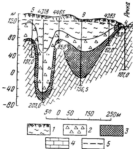
Рис. 43. Широтный геологический разрез карстово-эрозионной депрессии в районе Алапаевского железорудного месторождения. Составила Л. С. Архангельская по материалам Н. И. Евсева
