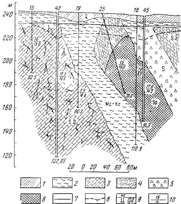
Рис. 42. Гидрогеологический разрез Быньговской водоносной зоны. По данным К. А. Костиной
