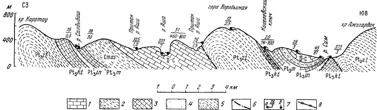
Рис. 37. Гидрогеологический разрез района хр. Каратау. Составили А. С. Веретенникова и Н. С. Анисимова по материалам В. Т. Брок и Н. А. Возжениковой
