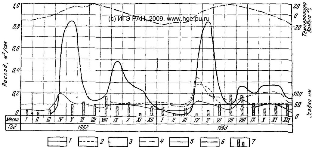
Рис. 26. График изменения среднемесячных расходов родников в контакте кобленцских и жединских известняков в Нижне-Сергинской синклинали
