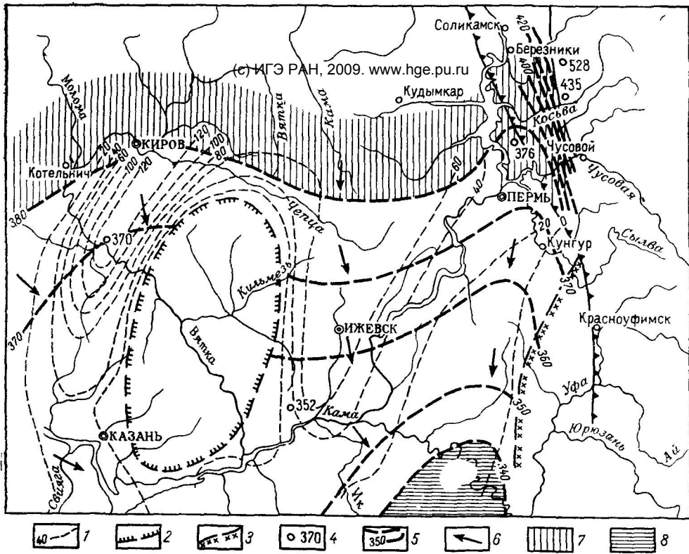
Рис. 16. Схематическая карта пьезометрической поверхности поверхности пластовых вод терригенных толщ верхнего девона. По В. И. Вещезероу и Б. М. Козлову, 1959 г.
