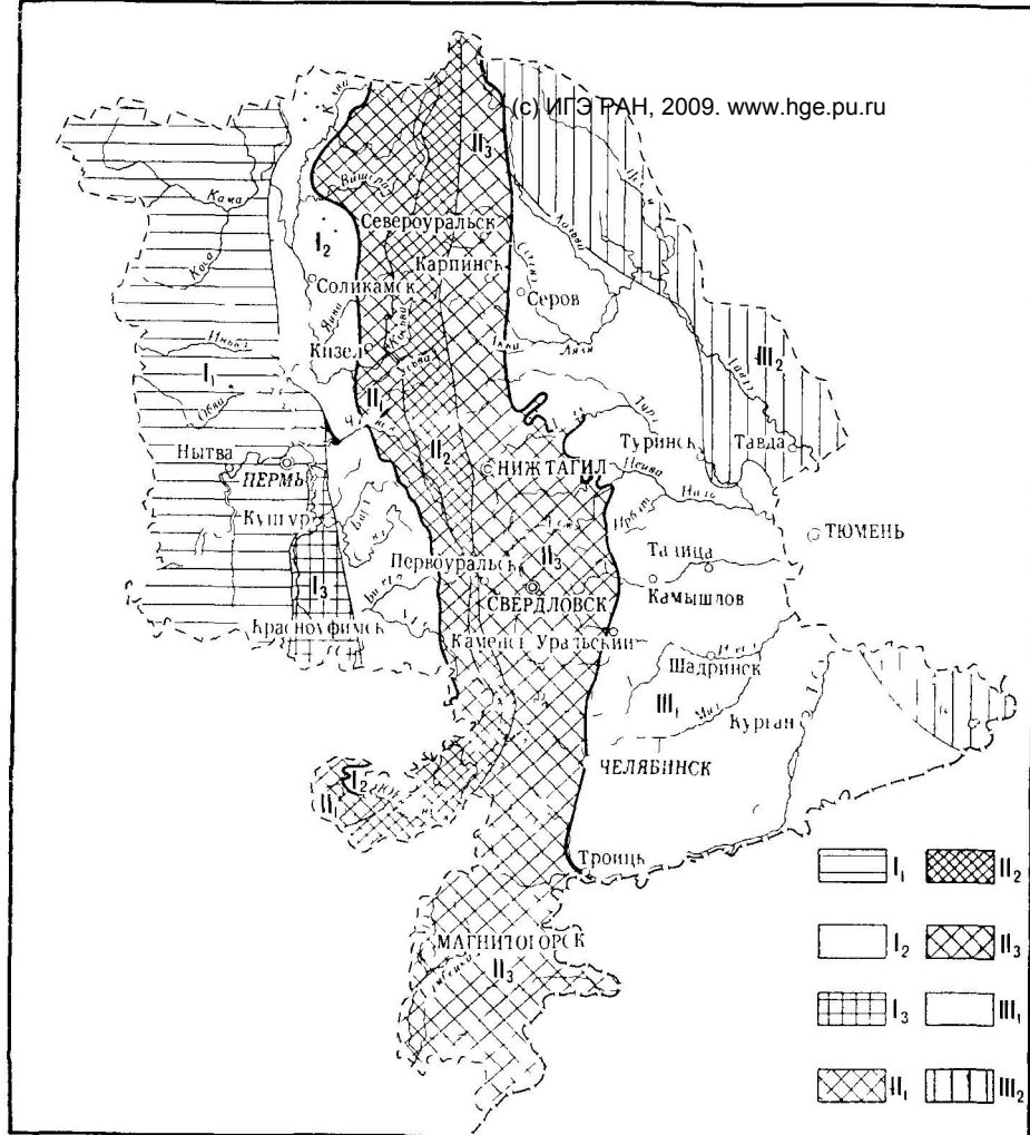
Рис. 7. Схема гидрогеологического районирования. Составили В. И. Антипин, А. С. Верегеникова, В. Ф. Прейс
