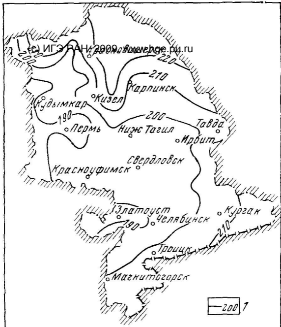
Рис 4 Схема средних многолетних глубин сезонного промерзания глинистых грунтов Урала
