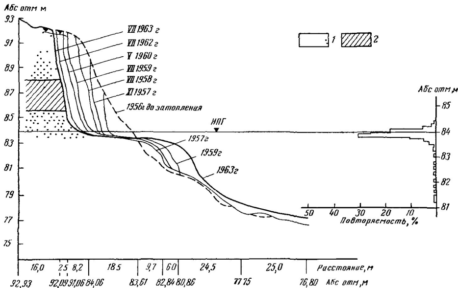
Рис. 108 Профиль берега на участке Андроновое на Горьковском водохранилище 1 — песок, 2 — суглинок
