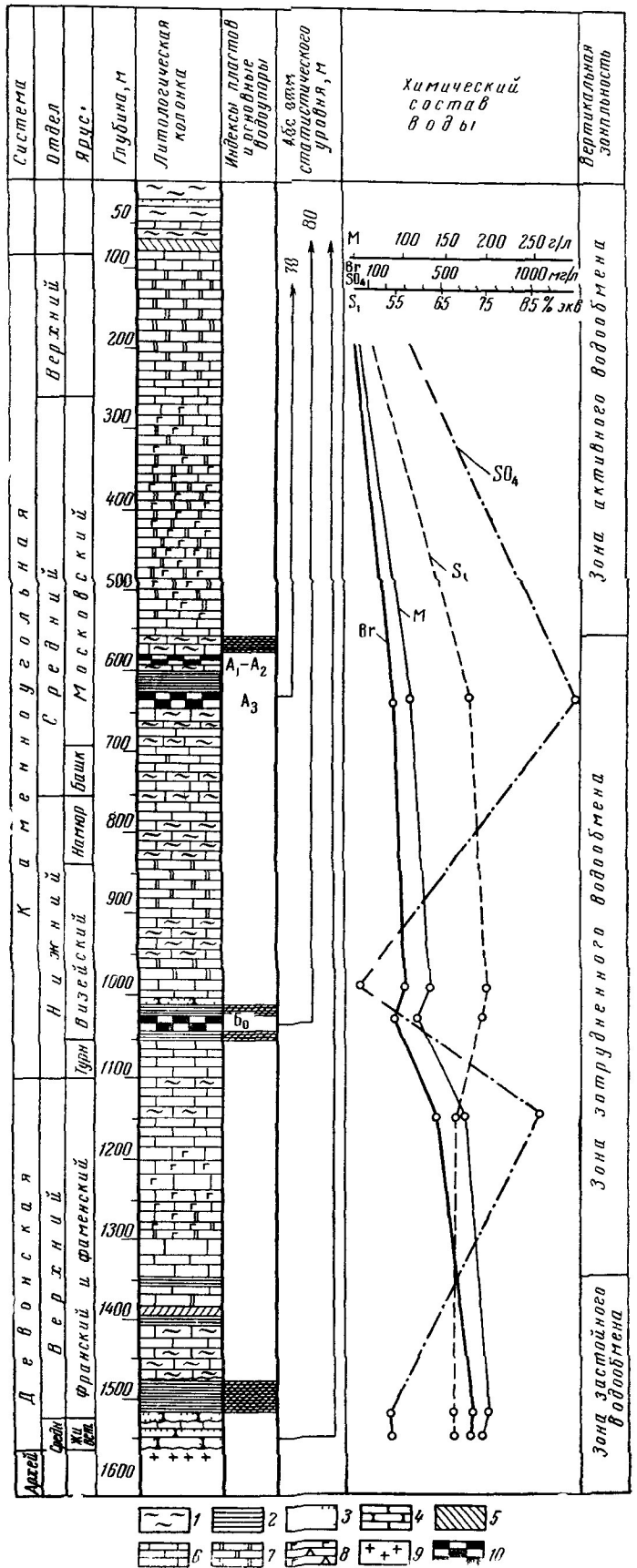
Рис. 86. Сводный гидрогеологический разрез Сызранского месторождения
