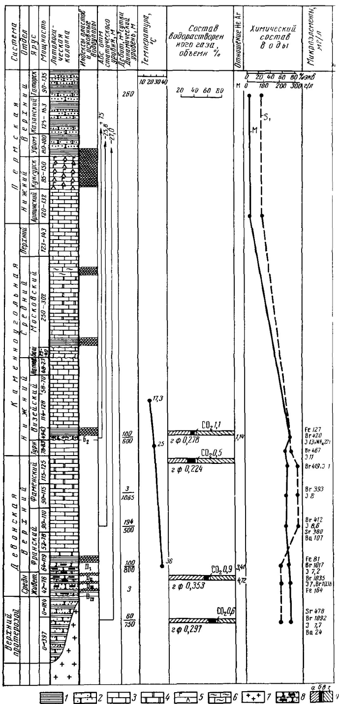
Рис. 82. Сводный гидрогеологический разрез Бавлинского месторождения 1 — аргиллиты; 2 — песчаники; 3 — известняки; 4 — доломиты; 5 — гипсы, ангидриты; 6 — глинистые известняки; 7 — кристаллический фундамент; 8 — нефтеносные породы; 9 — состав водорастворенного газа в объем. %: a — \text{CH}_4 ; b — \text{C}_n\text{H}_{2n+2} ; v — кислые газы ( \text{CO}_2 , \text{H}_2\text{S} , \text{H}_2 ); z — \text{N}_2 + редкие; г. ф. — газовый фактор в л/л
