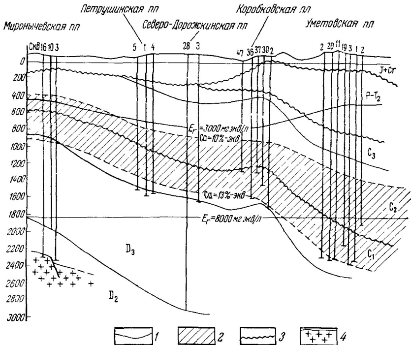
рис 77 Гидрогеохимический профиль по центральной части Волгоградской области 1 — границы минерализации, 2 — содержание кальция, 3 — стратиграфические границы, 4 — кристаллический фундамент
