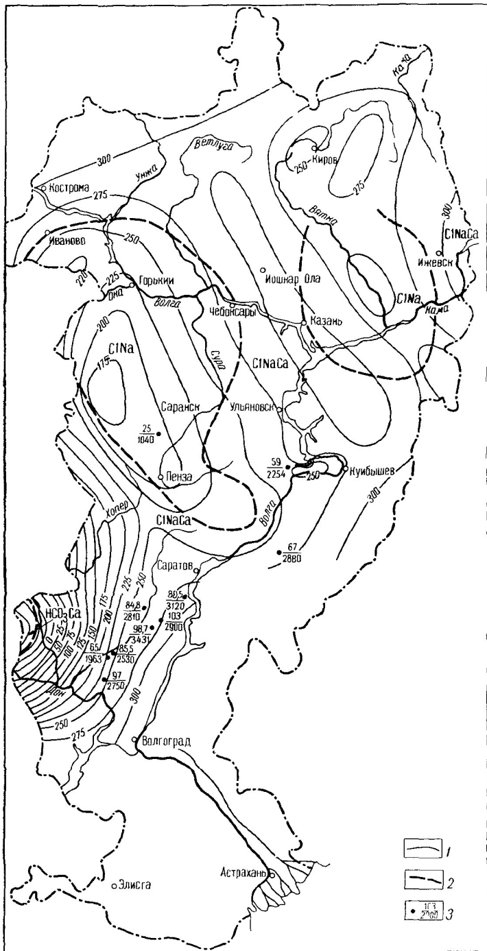
Рис. 76. Схема состава и минерализации термальных вод и рассолов на поверхности кристаллического фундамента. Составили Т. П. Афанасьев и Н. Д. Козлова 1 — изолинии минерализации в г/л 2 — граница гидрохимической зоны подземных вод; 3 — скважина (цифры в числителе — температура воды в °С, в знаменателе — глубина отбора пробы в м)
