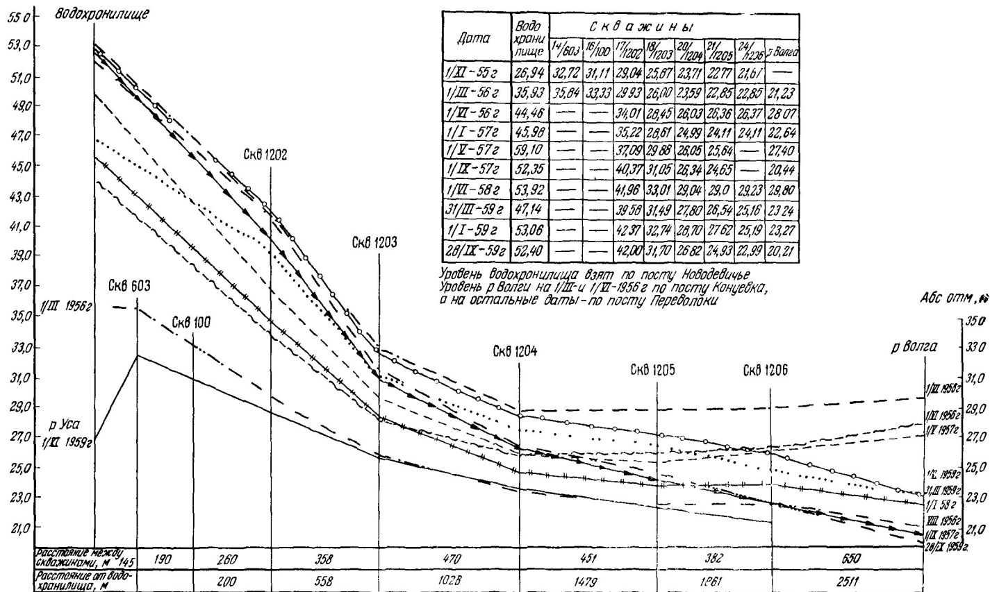
Рис. 57. Изменения уровня подземных вод на Волго-Усинском водоразделе под воздействием Куйбышевского водохранилища (Переволоцкий гидрогеологический пост)
