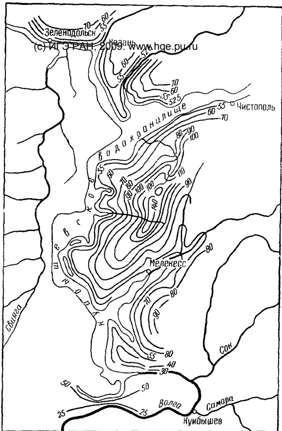
Рис 56 Схема гидроизогипс левобережья Куйбышевского водохранилища (лето 1958 г)
