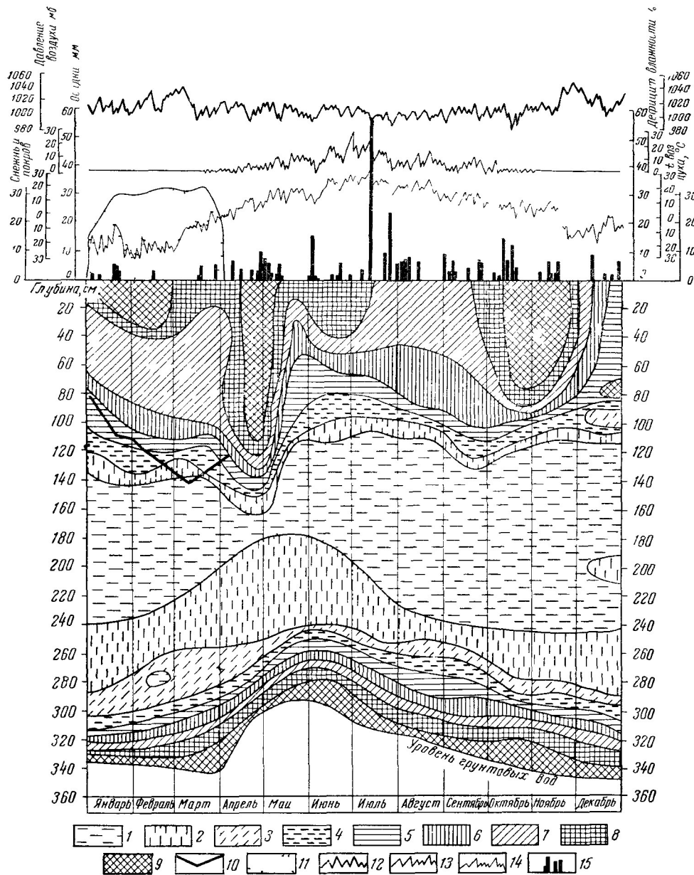
Рис 51 График гидроизоплет зоны аэрации в районе г Мелекесса за 1954 г
