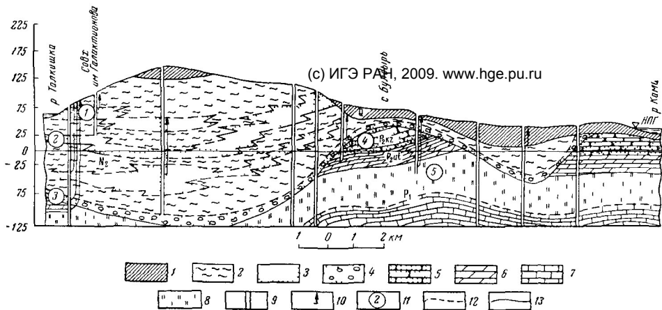
Рис. 31. Гидрогеологический разрез левобережья р. Камы по линии расположения селений Талкишка — Булдырь Чистопольского района
