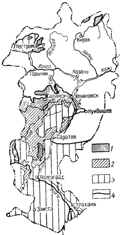
Рис. 17. Распространение меловых отложений
