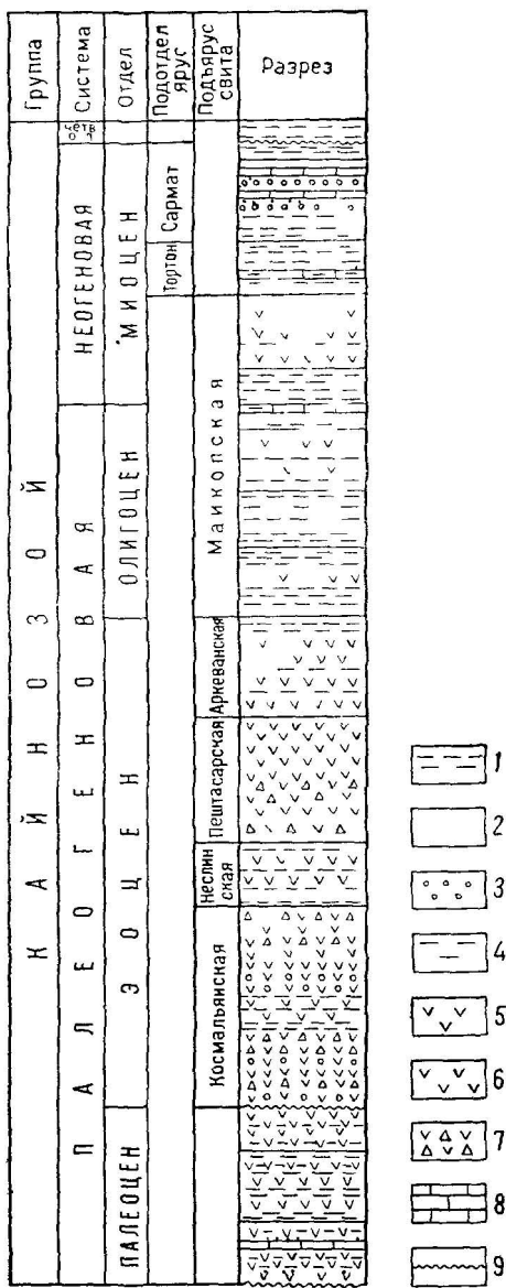
Рис. 9. Сводная стратиграфическая колонка гидрогеологического района Талыша и Ленкоранской низменности
