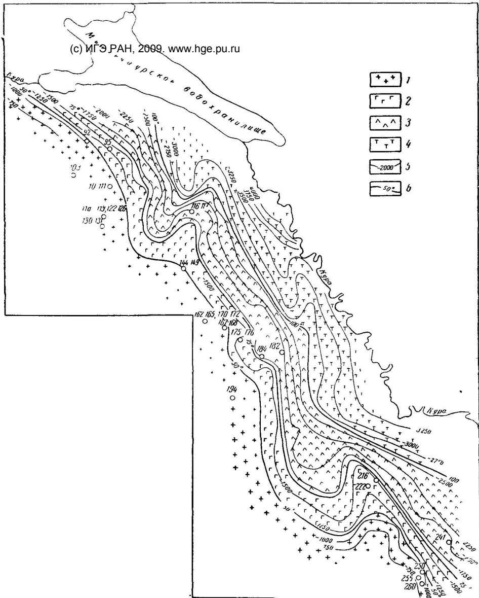
Рис. 31. Схематическая геотермическая карта по кровле майкопских отложений ( Pg+N_1 ). Геотемпературные зоны 1 — 20–50°; 2 — 50–75°; 3 — 75–100°; 4 — 100° и более; 5 — стратотипы по кровле майкопских отложений; 6 — границы геотемпературных зон
