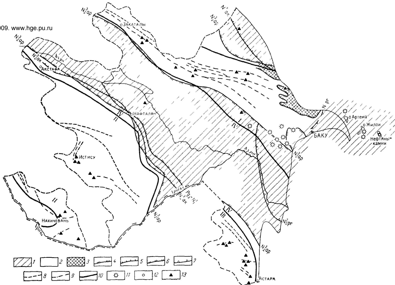
Рис. 29. Схематическая карта распространения термальных вод Азербайджанской ССР
