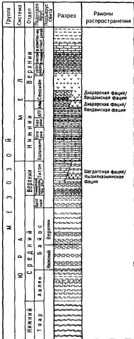
Рис. 2. Сводная стратиграфическая колонка гидрогеологического района Большого Кавказа а — мезозой, б — кайнозой
